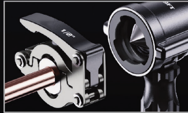
Eksantrik havşa açma konisi
