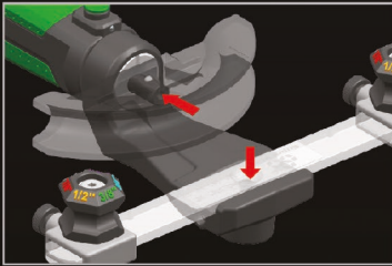
Bükme kalıbı ve universal traversin hızlı montajı
